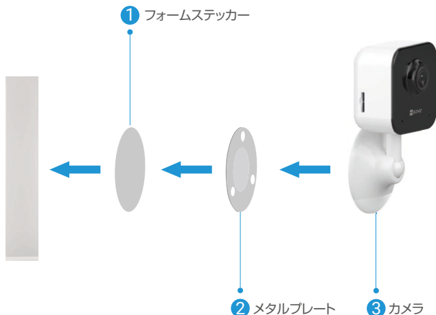
図 1 フォームステッカーによる取り付け
