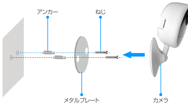
図2 ねじによる取り付け
